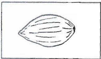
mamão
